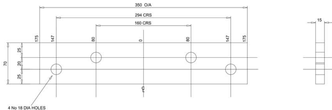
ITEM 10 70 x 15 x 350 LONG - FLAT BAR SCALE 1 : 2
