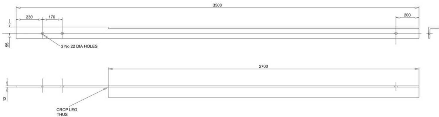
ITEM 9 100 x 100 x 12 ANGLE - 3500 LONG SCALE 1 : 10
